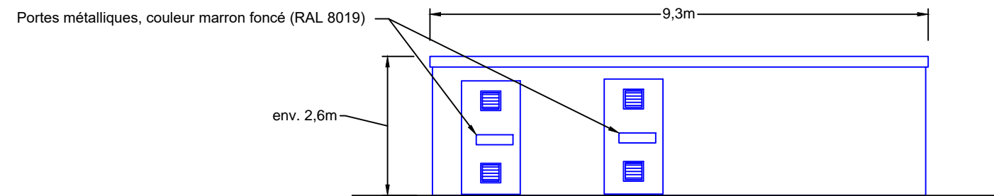
Facade nord
