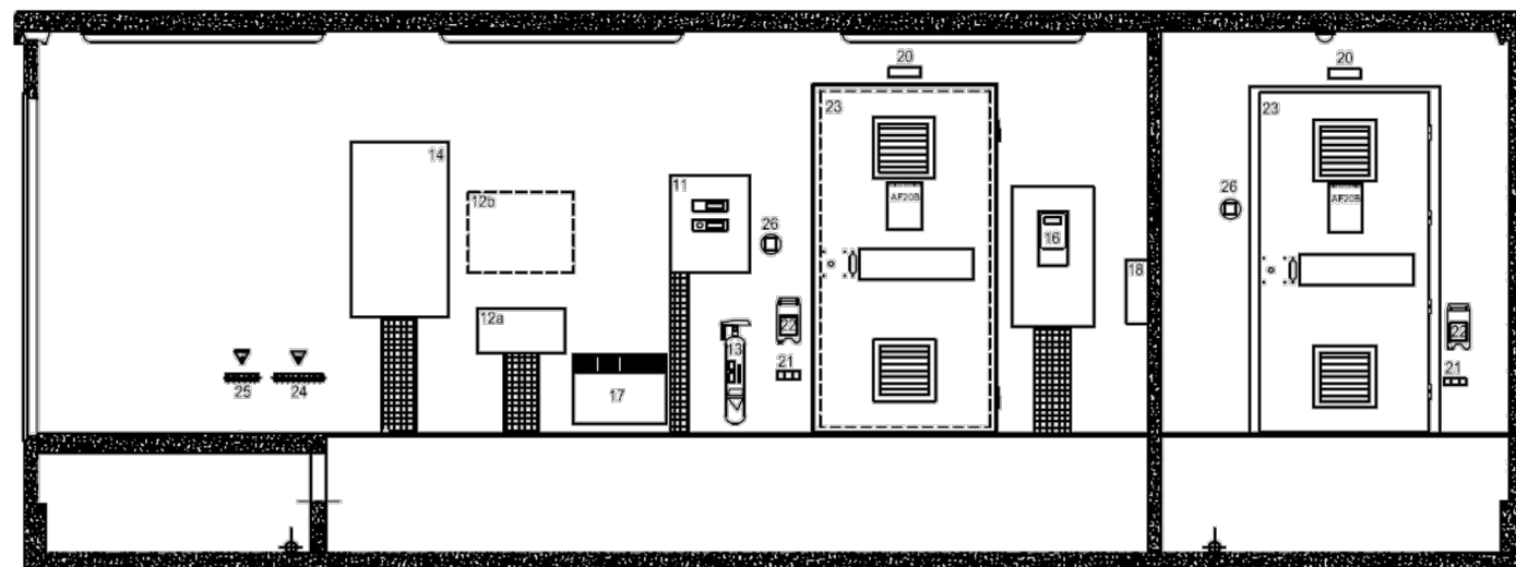
COUPE B-B
